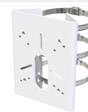
A02 V2 Pole Mount
