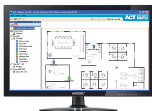
Site Maps
